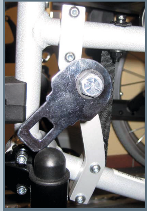
Zwei hintere Kraftknotensysteme mit jeweils einer genormten Schwerlastöse für Spannretractor. Der Beckengurt ist bereits fest montiert.
