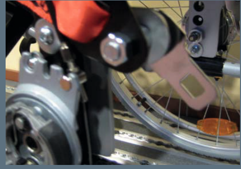
Zwei vordere Kraftknotensysteme mit jeweils einer Schwerlastöse für Spannretractor oder Statikgurt.
